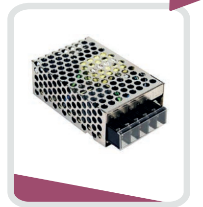
VEL RS-25-24 ALIMENTATION COMPACTE A DECOUPAGE 1 SORTIE 25W 24V
